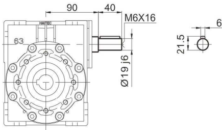
Output flange 输出法兰
